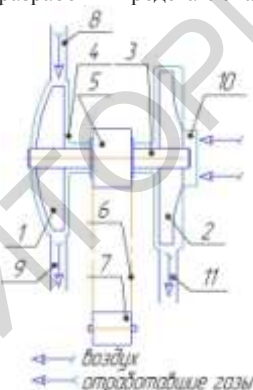
Рисунок – Турбокомпрессор двигателя внутреннего сгорания
