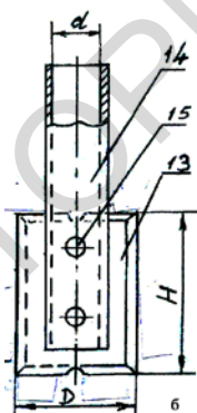
Рисунок 2 – Схема почвенной фрезы
