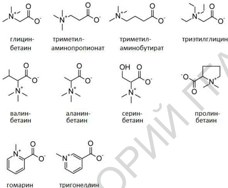
Рисунок 1 – Гомологи глицин-бетаина
