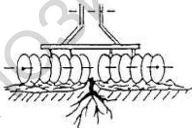
Рисунок 2 – Схема разокучивания рядов хмеля дисковой бороной
