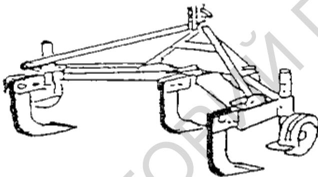
Рисунок 9 – Рыхлитель почвы в междурядьях хмеля
