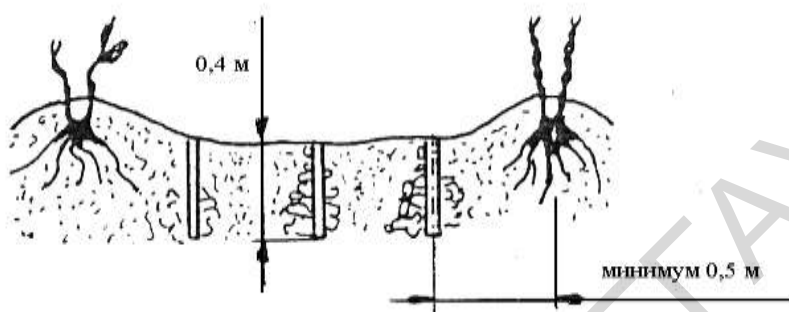
Рисунок 10 – Схема глубокого рыхления почвы в междурядьях хмеля
