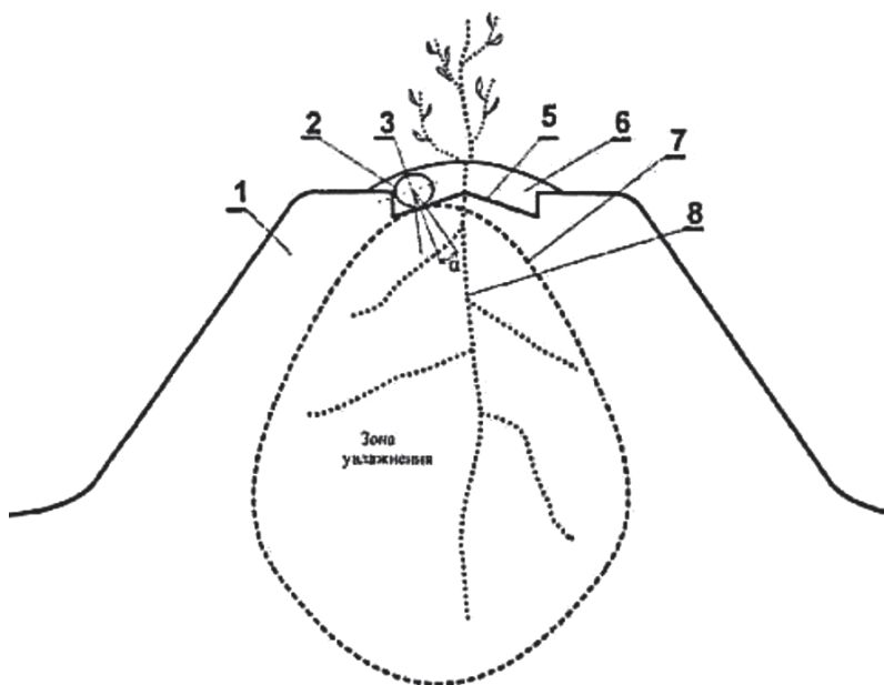
Рис. 10. Схема укладки поливного шланга на гребне
